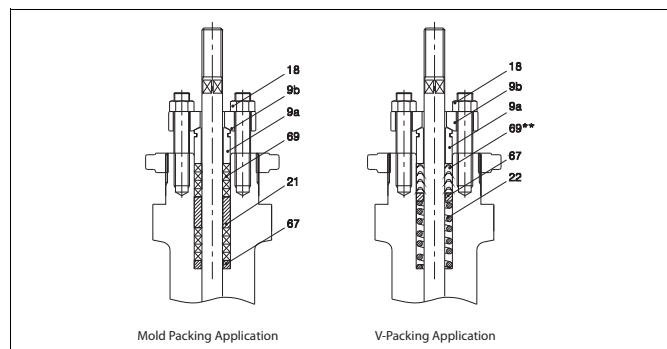
Fig. 7 Gland packing
